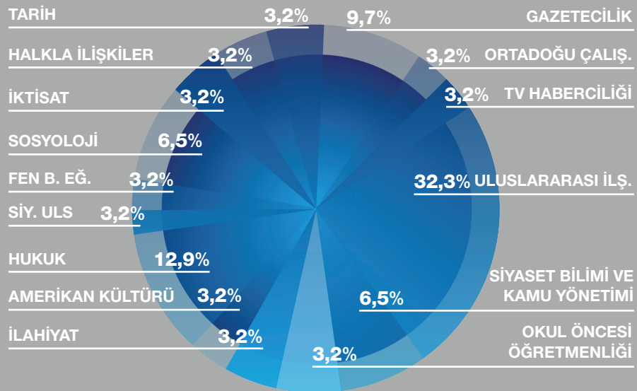
ŞEKİL 23 | Katılımcıların bölümleri
